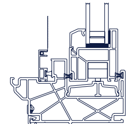
1" Mounting Fin Set-back
